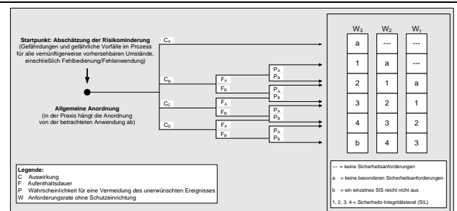
Bild 3: Risikograph
