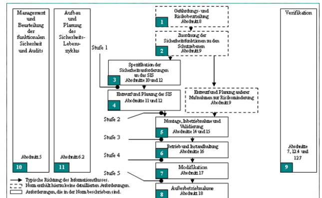
Bild 1: Sicherheitslebenszyklus (IEC/ DIN EN 61511)
